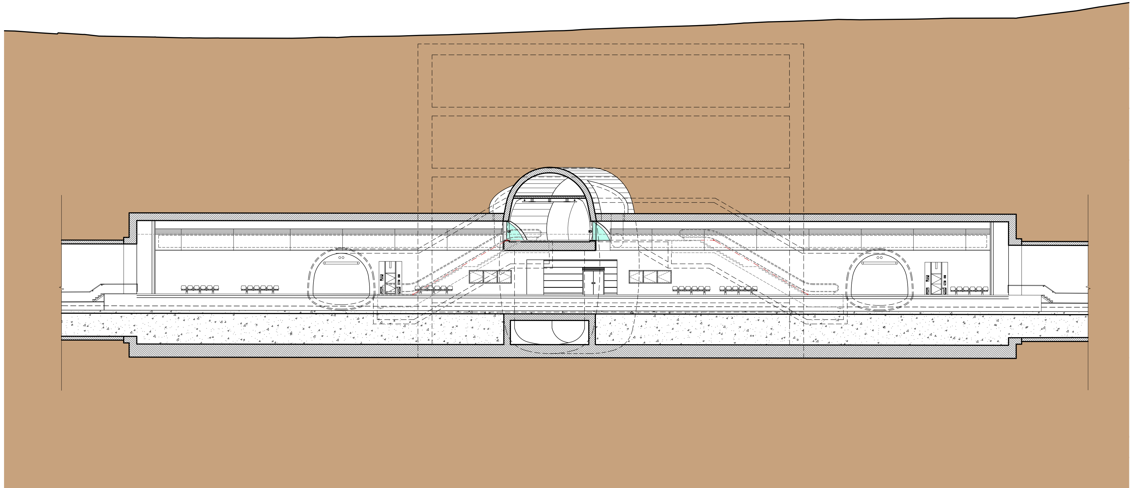
TOMH A-A
