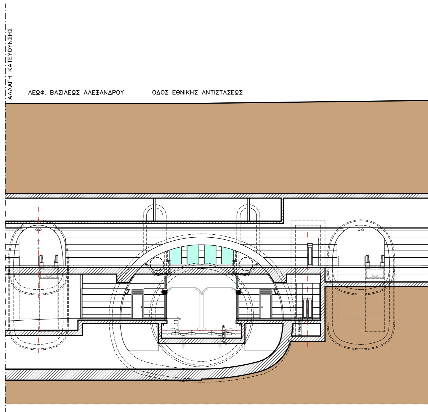
ΤΟΜΗ C1—C1
