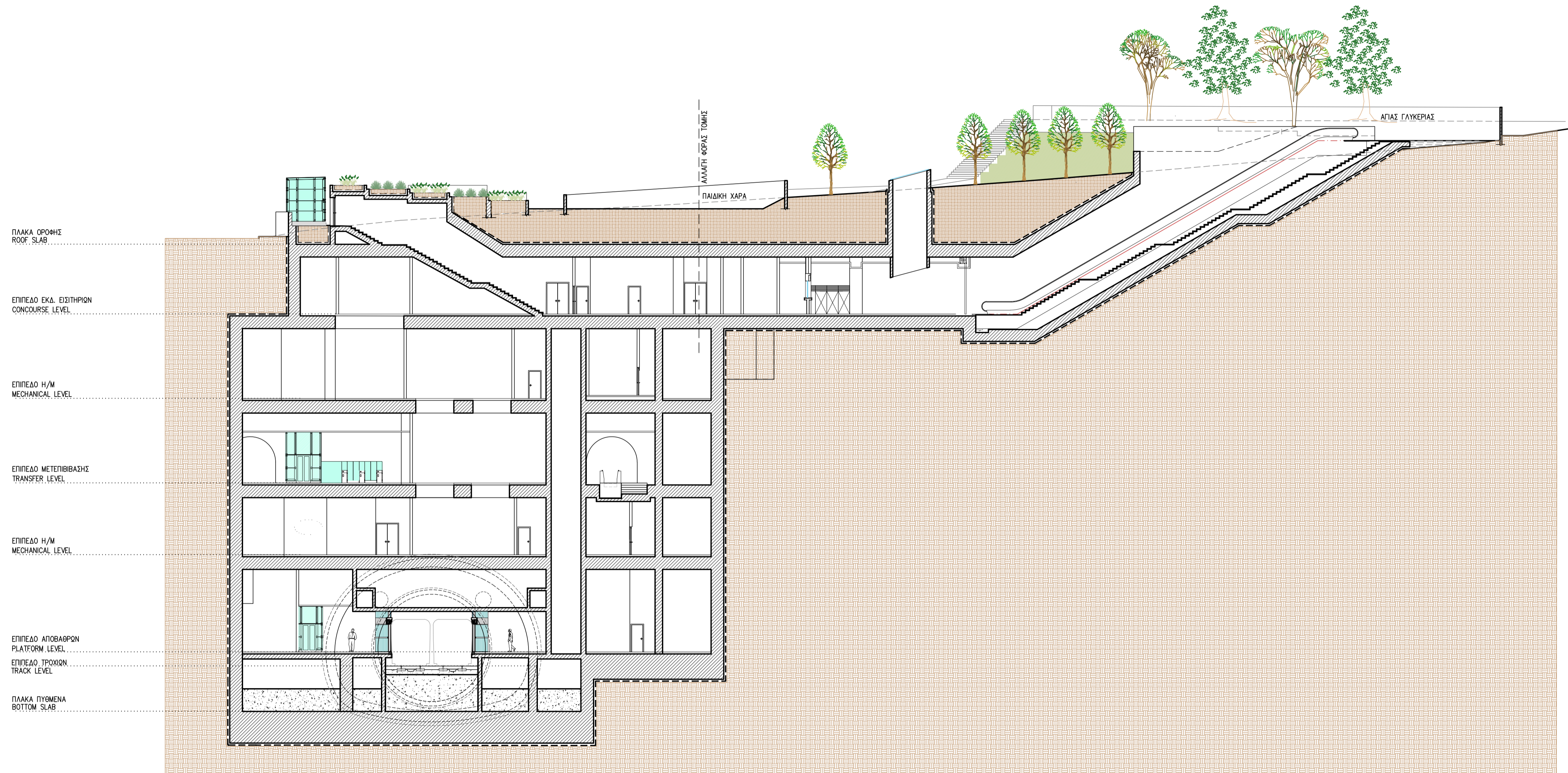
ΤΟΜΗ Β-Β
